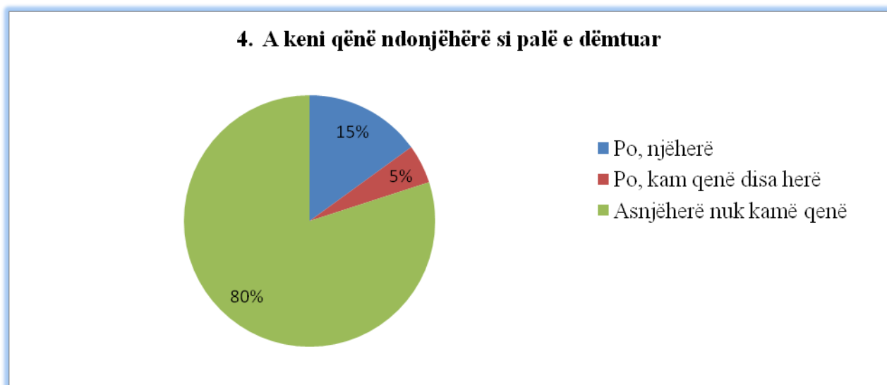
Grafikoni nr.4
